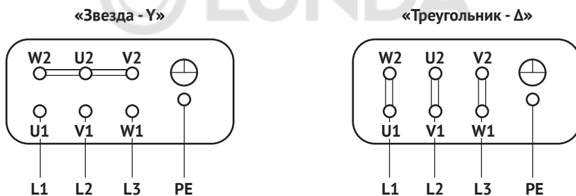
Рисунок 4 – Схема подключения электродвигателя
