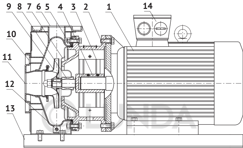
Рисунок 2 – Общий вид и конструкция насоса
