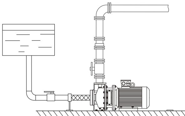
Рисунок 5 – Насос установлен ниже уровня перекачиваемой жидкости
