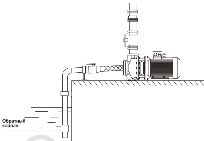
Рисунок 6 – Насос установлен выше уровня перекачиваемой жидкости
