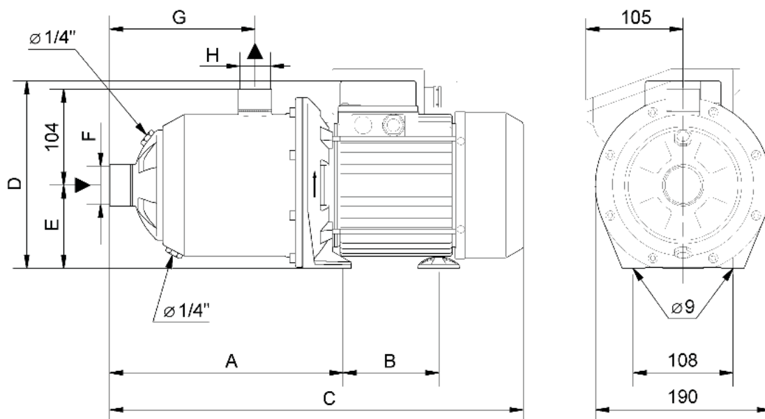
Рисунок 3. Габаритный чертеж
