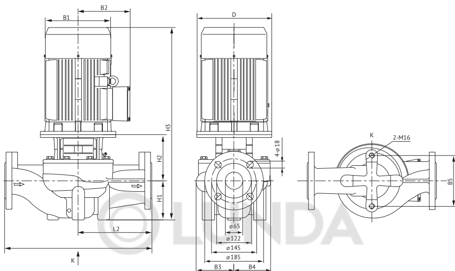
Рисунок 4 – Насосы SVH 65
