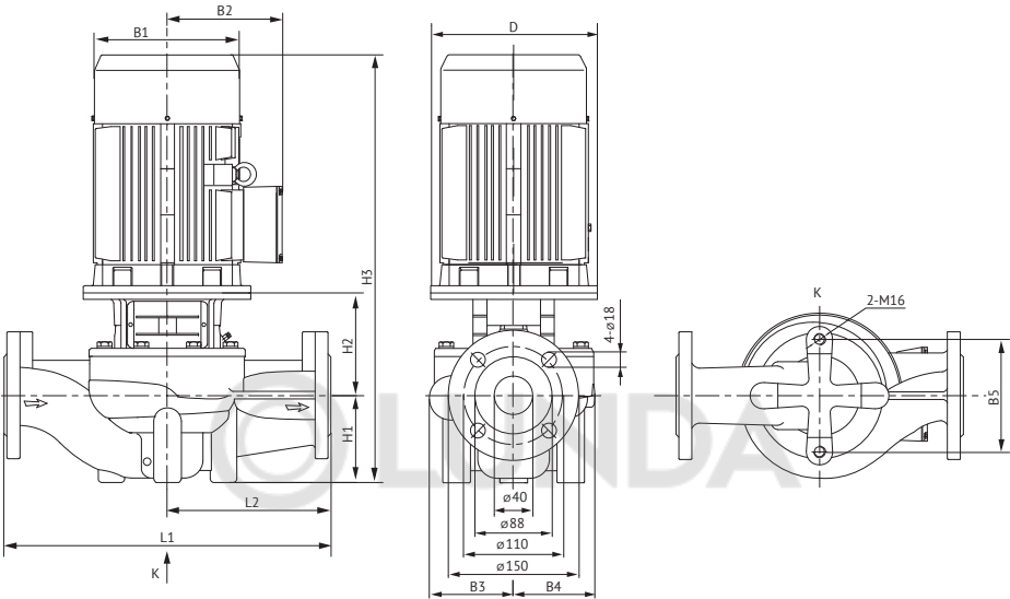
Рисунок 2 – Насосы SVH 40
