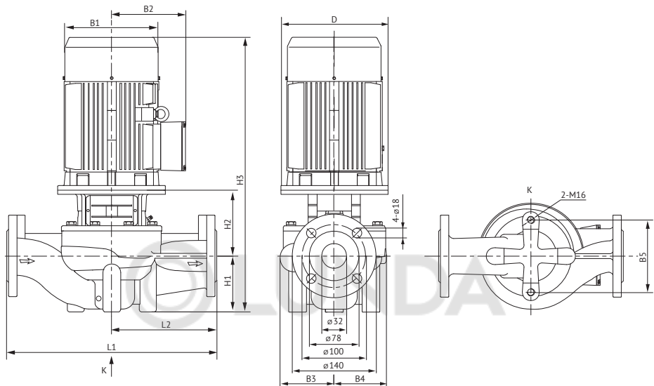
Рисунок 1 – Насосы SVH 32
