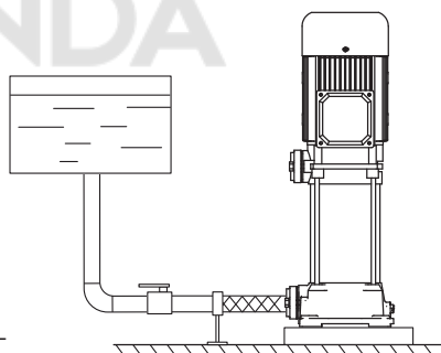
Рисунок 7 – Насос установлен ниже уровня перекачиваемой жидкости
