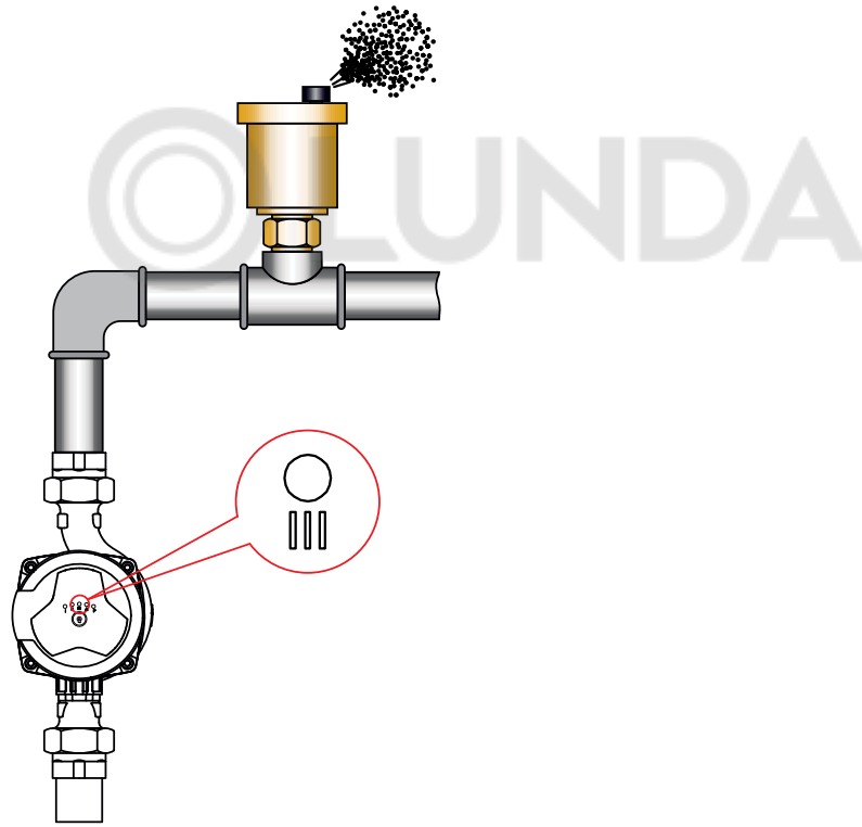
Рис.2 Удаление воздуха из корпуса насоса.
