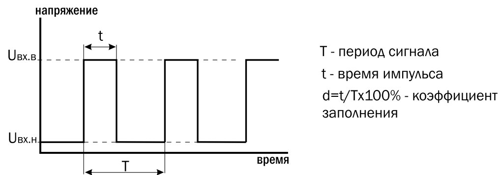
Рис.13 Характеристики ШИМ-сигнала.
