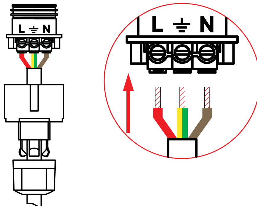
Рис.7 Схема подключения насоса.
