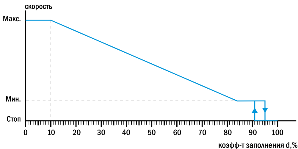
Рис.14 Зависимость скорости от коэффициента заполнения.
