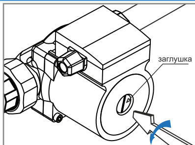
Рис.6. Удаление воздуха из корпуса насоса.
