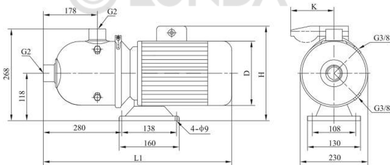
Габаритно-присоединительные размеры
