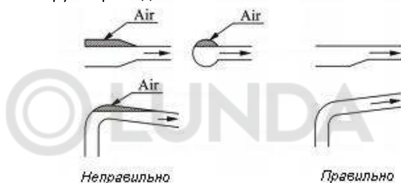
Рис. 3 Схемы расположения впускного трубопровода
