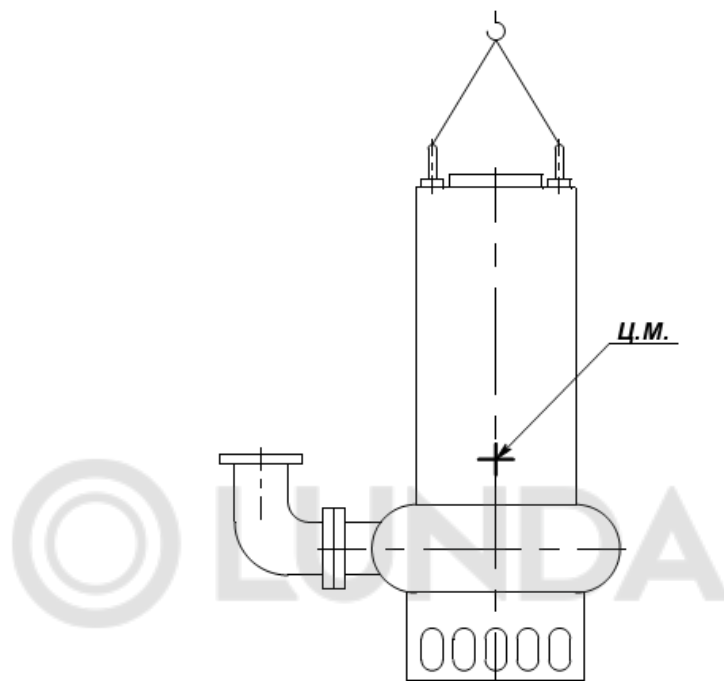
Рис. 2 Схема строповки насоса без тары
