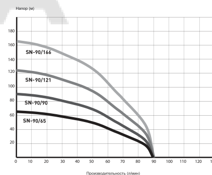
Расходно-напорные характеристики для насосов SN-90/65, 90/90, 90/121, 90/166
