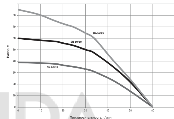
Расходно-напорные характеристики насосов с диаметром 3,5"
