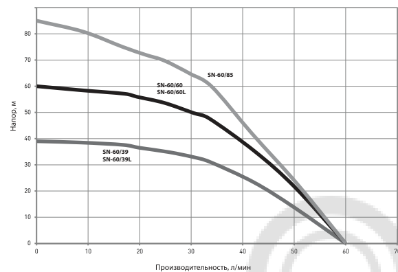
Расходно-напорные характеристики насосов с диаметром 3,5"
