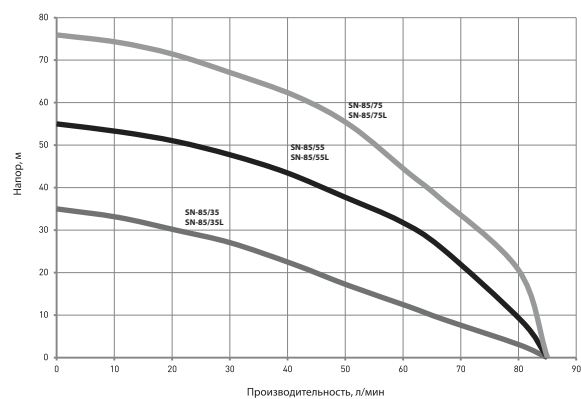
Расходно-напорные характеристики насосов с диаметром 4"
