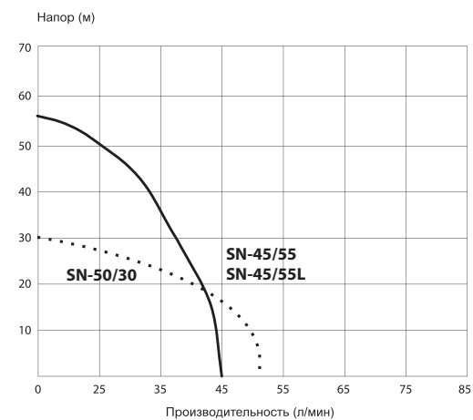
Расходно-напорные характеристики для насосов SN-45/55, SN-45/55L и SN-50/30
