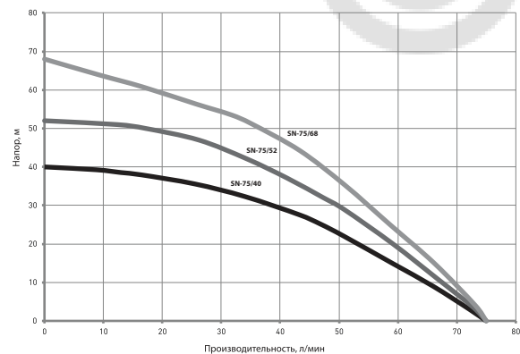
Расходно-напорные характеристики насосов с диаметром 4"
