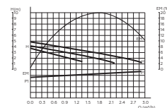
Rommer 32/40-180
