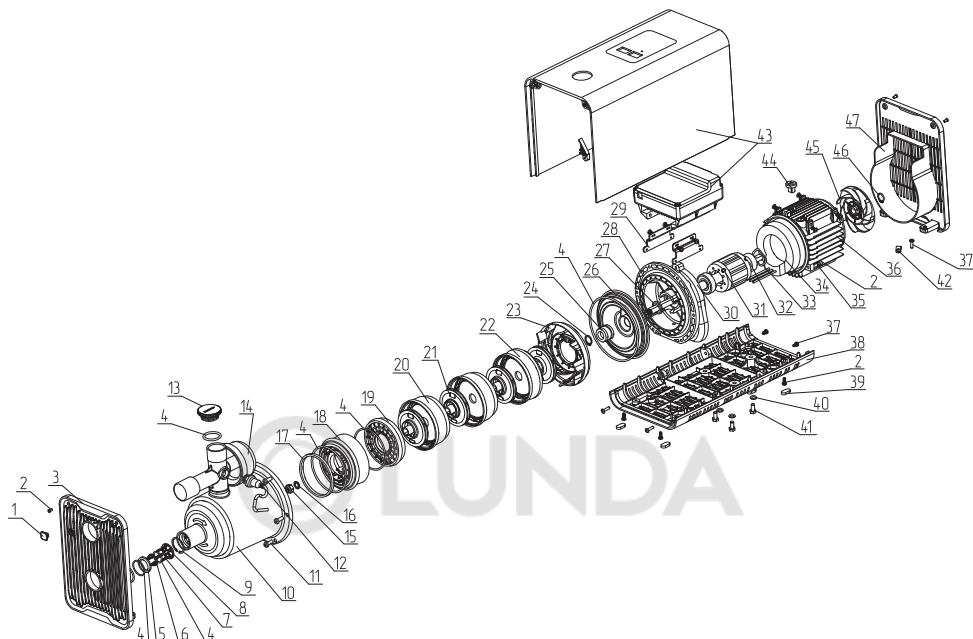
Рис.2 Устройство насосной станции ZOTA LaScala
