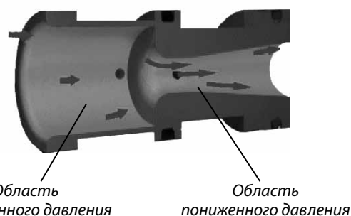
Рис. 36. Конструкция измерительной диафрагмы клапана БРОЕН Dynamic
