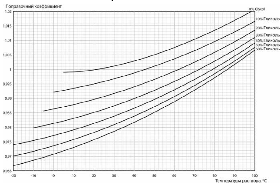
Рис.67. График зависимости поправочного коэффициента для водного раствора этиленгликоля от температуры и концентрации
