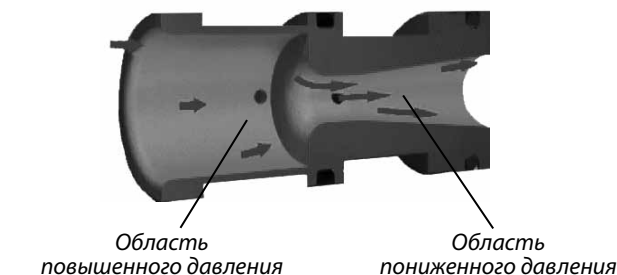
Рис.8 Конструкция измерительной диафрагмы клапана БРОЕН Venturi
