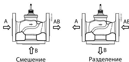
Рис.1. Работа клапана на смешение потоков или разделение потока
