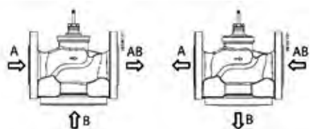
Рис. 1. Смешение или разделение потоков.
