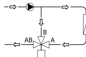
Рис.3. Смесительный клапан на разделение потока
