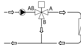
Рис.4. Разделительный клапан на разделение потока
