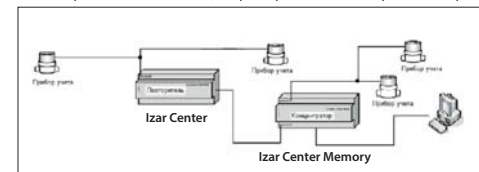
Схема передачи данных с концентратора на компьютер диспетчера
