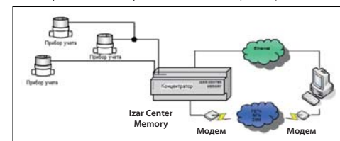
Схема передачи данных через модем или Ethernet (Internet)
