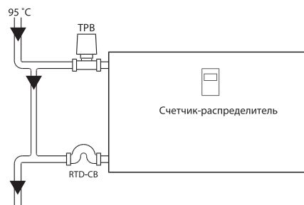
RTD-CB в однетрубной системе отопления с замыкающими участками, терморегуляторами и счетчиками-распределителями
