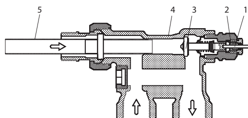
б — RA 15/6T для одноконтурной системы отопления с патрубками для трубопроводов \frac{1}{2} "
