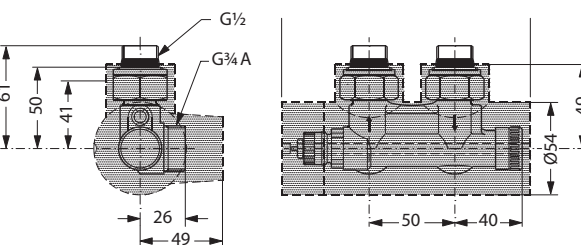
Гарнитура VHS с тыльным подключением. Радиаторное присоединение 1/2" или 3/4"
