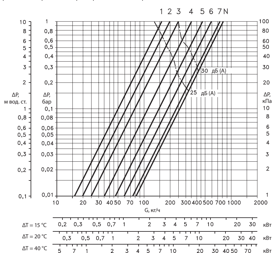
Диаграмма для определения предварительной настройки клапана RA-N 20 UK
