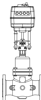
AME 65x + VFG(S) 2 + адаптер 065B3525 ( D_y = 15-65 мм) 065B3526 ( D_y = 80-125 мм) 065B3527 ( D_y = 150-250 мм)
