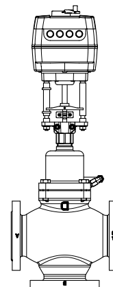
AME 65x + VFG 33 + адаптер 065B3525 ( D_y = 25-65 мм) 065B3526 ( D_y = 80-125 мм) 065B3527 ( D_y = 150-250 мм)
