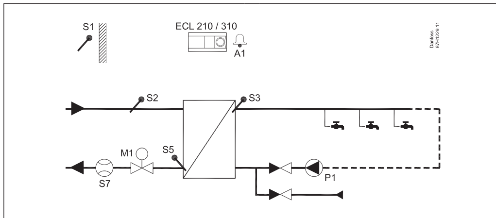
A217.3, пр. с: Нагрев ГВС по требованию ( датчик протока). С циркуляцией или без.
