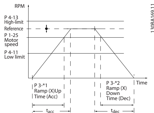
Рисунок 3.17 Изменение скор. 1
