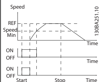
Рисунок 3.24 Принцип управления обходным клапаном
