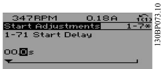
Рисунок 2.19 Выбор цифры
