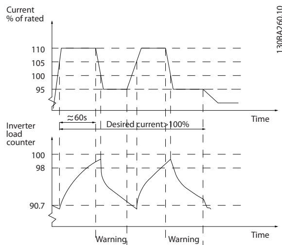
Рисунок 3.44 Выходной ток в условиях перегрузки
