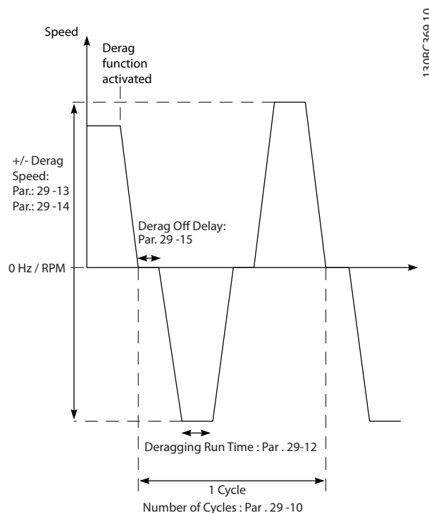
Рисунок 3.85 Функция очистки
