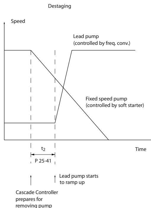
Рисунок 3.77 Выключение
