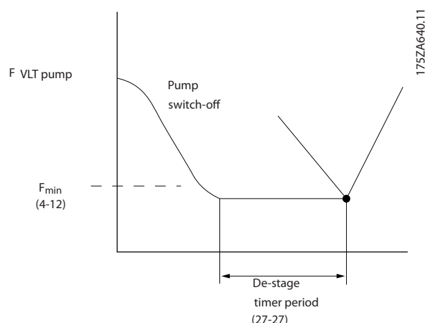
Рисунок 3.75 Задержка выключения
