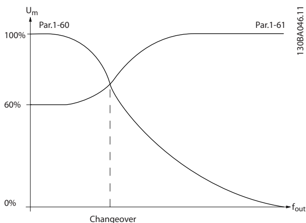
Рисунок 3.10 Компенсация нагрузки на низк.скорости
