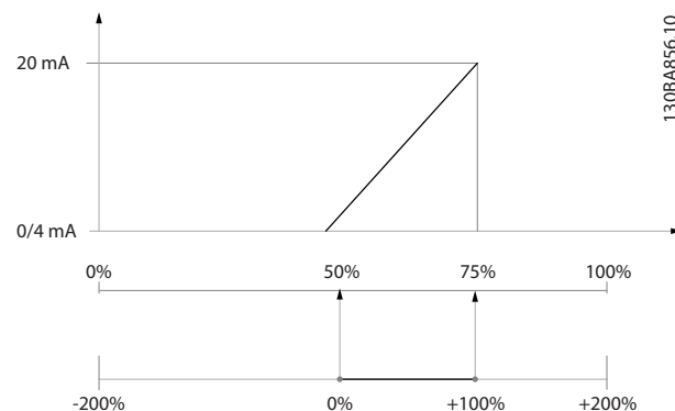
Рисунок 3.34 Пример 2
