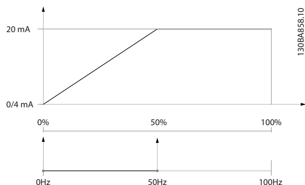
Рисунок 3.33 Пример 1
