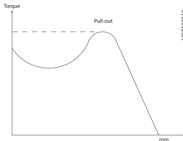
Рисунок 1.1 Момент опрокидывания
