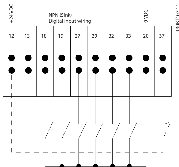
Рисунок 1.4 NPN (сток)
