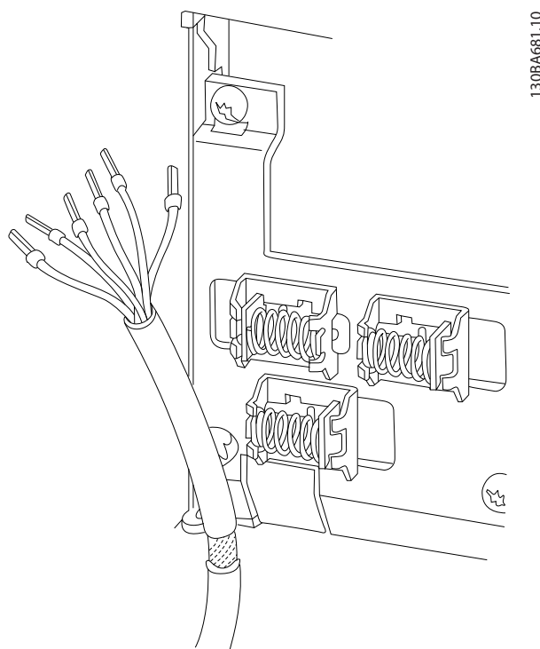
Рисунок 1.5 Заземление экранированных/защищенных кабелей управления
