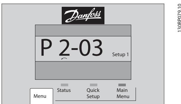
Рисунок 2.24 Главное меню/быстрая настройка
