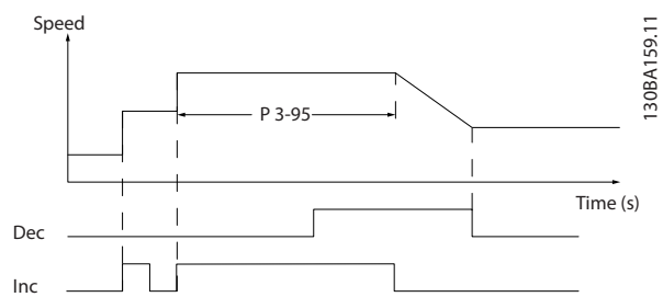
Рисунок 3.22 Задержка изменения скорости, случай 2
