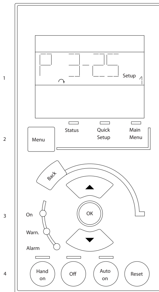
Рисунок 2.21 Кнопки LCP
