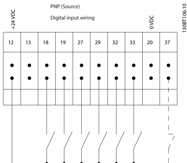
Рисунок 1.3 PNP (источник)
