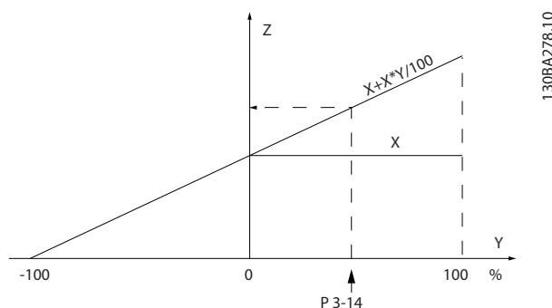
Рисунок 3.16 Фактическое задание
