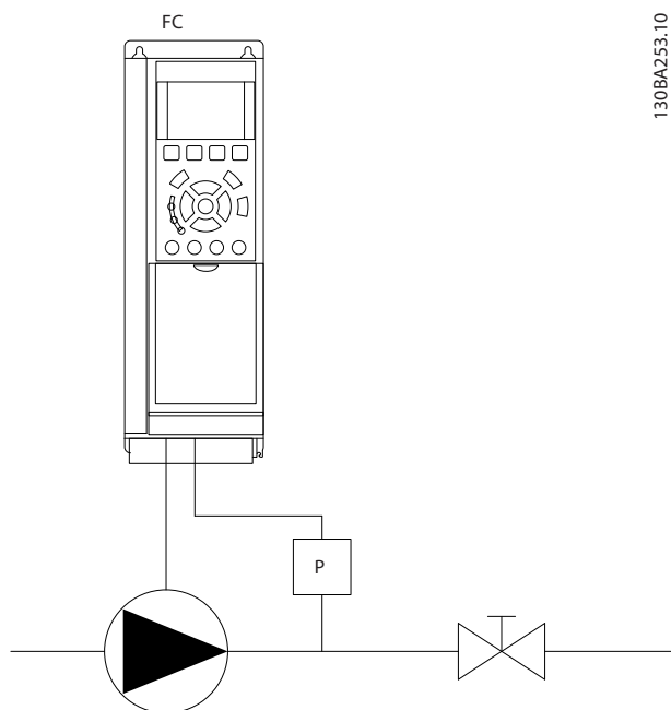
Рисунок 3.51 Схема обнаружения отсутствия потока
