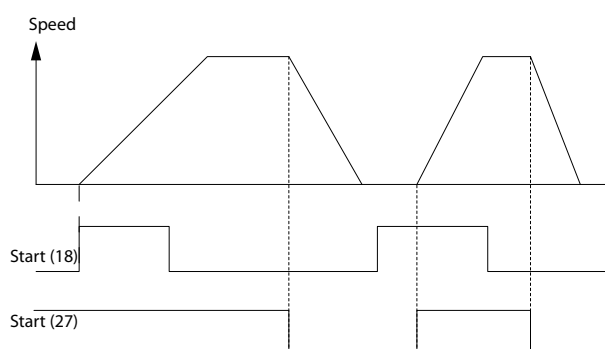
Рисунок 1.7 Импульсный пуск/останов
