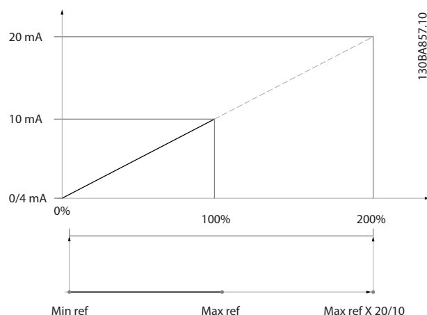
Рисунок 3.35 Пример 3
