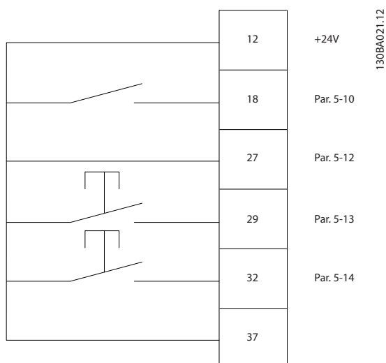
Рисунок 1.8 Увеличение/снижение скорости
