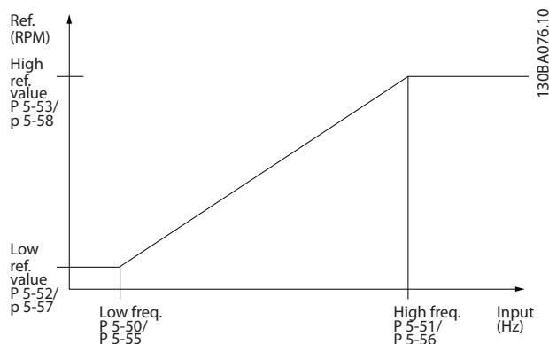
Рисунок 3.27 Импульсный вход
