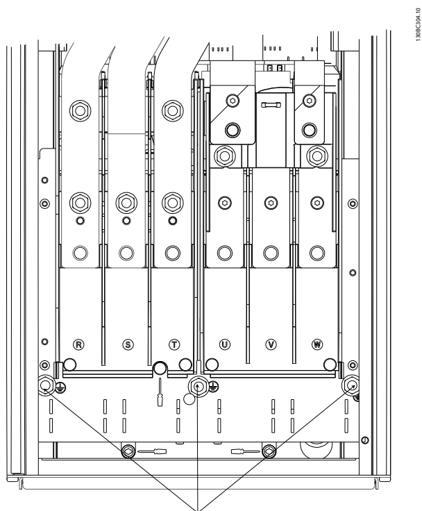
Рисунок 2.6 Заземление (зануление) для корпусов IP21/54.
