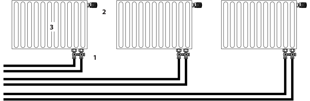
двухтрубная система (байпас закрыт)
