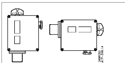
Рис. 1. Монтажное положение реле давления.
