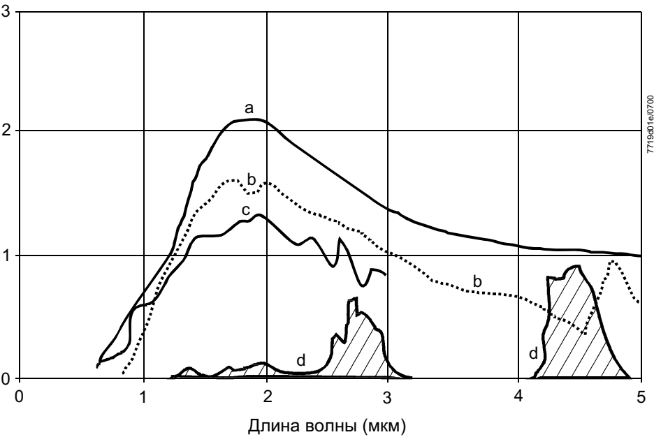
Спектральная эмиссия излучения светящегося и несветящегося пламени при 1,500 К (выписка из VDI Отчета по. 423, 1981).
