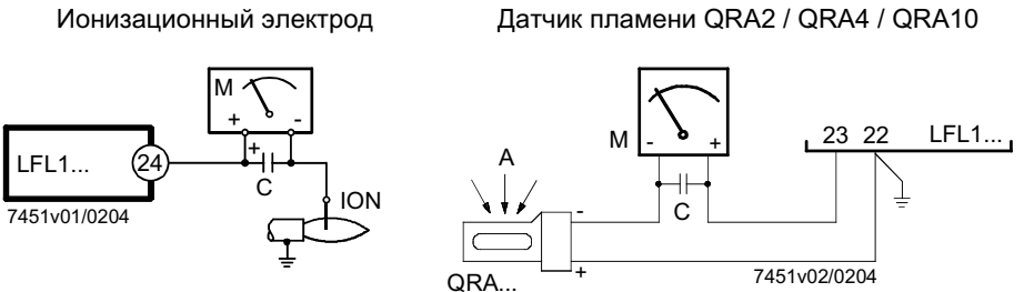
Схема измерения тока датчика
