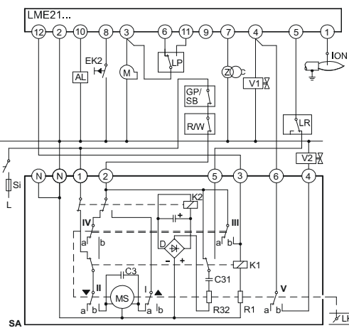
SQN91.140.../2-ступенчатое управление
