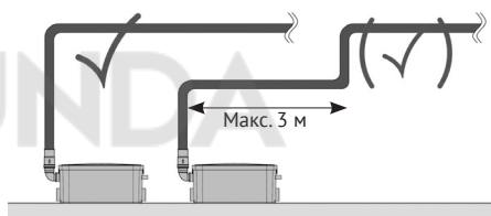
Рисунок 9 – Вертикальный участок напорного трубопровода
