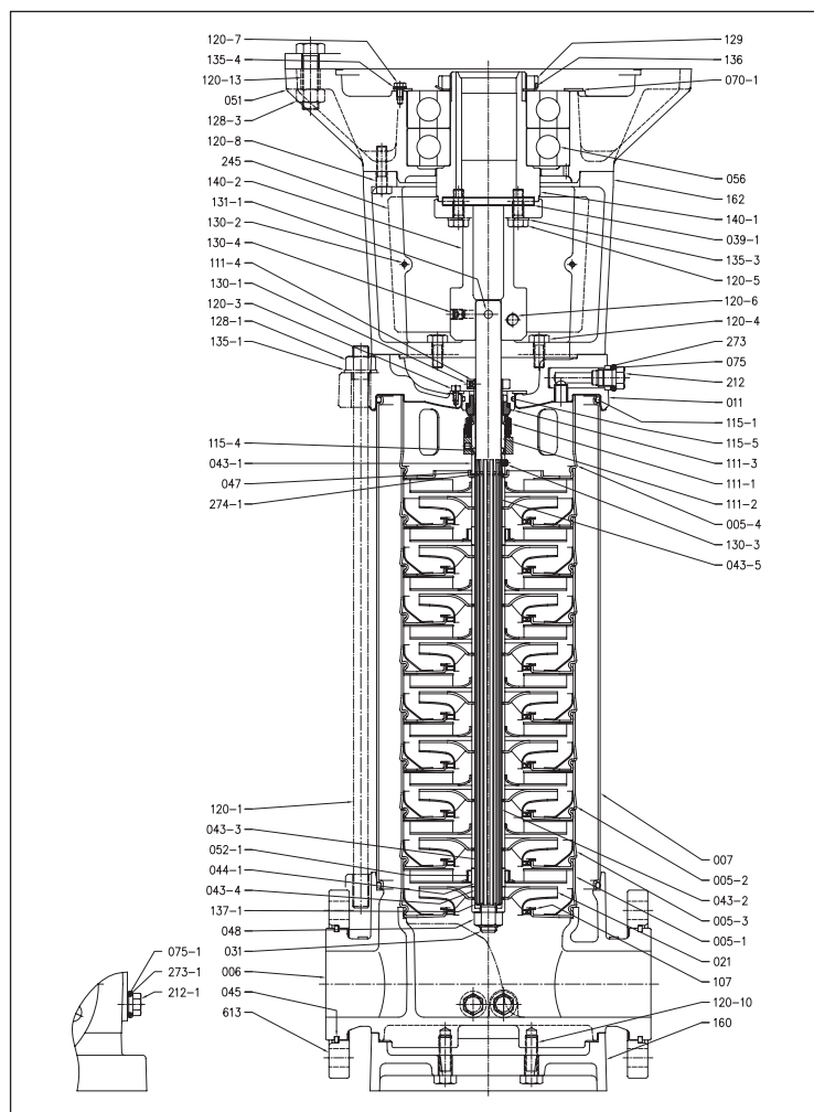
РАЗРЕЗ EVM(L) 32 Насос с двойным шариковым подшипником
