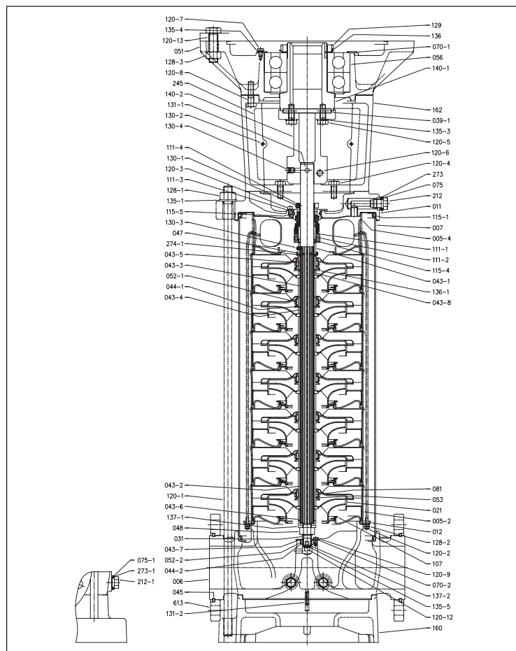
РАЗРЕЗ EVM(L) 45-64 Насос с двойным шариковым подшипником
