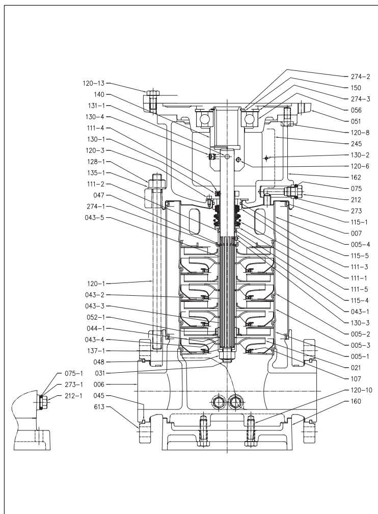
РАЗРЕЗ EVM(L) 32 Насос с одинарным шариковым подшипником
