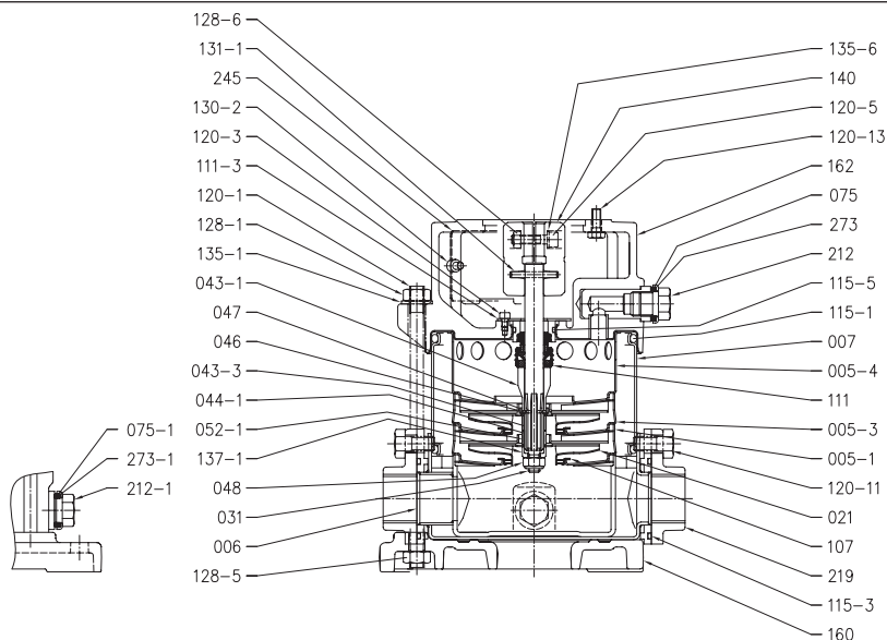
РАЗРЕЗ EVM(L) 3-18 Насос с одинарным шариковым подшипником
