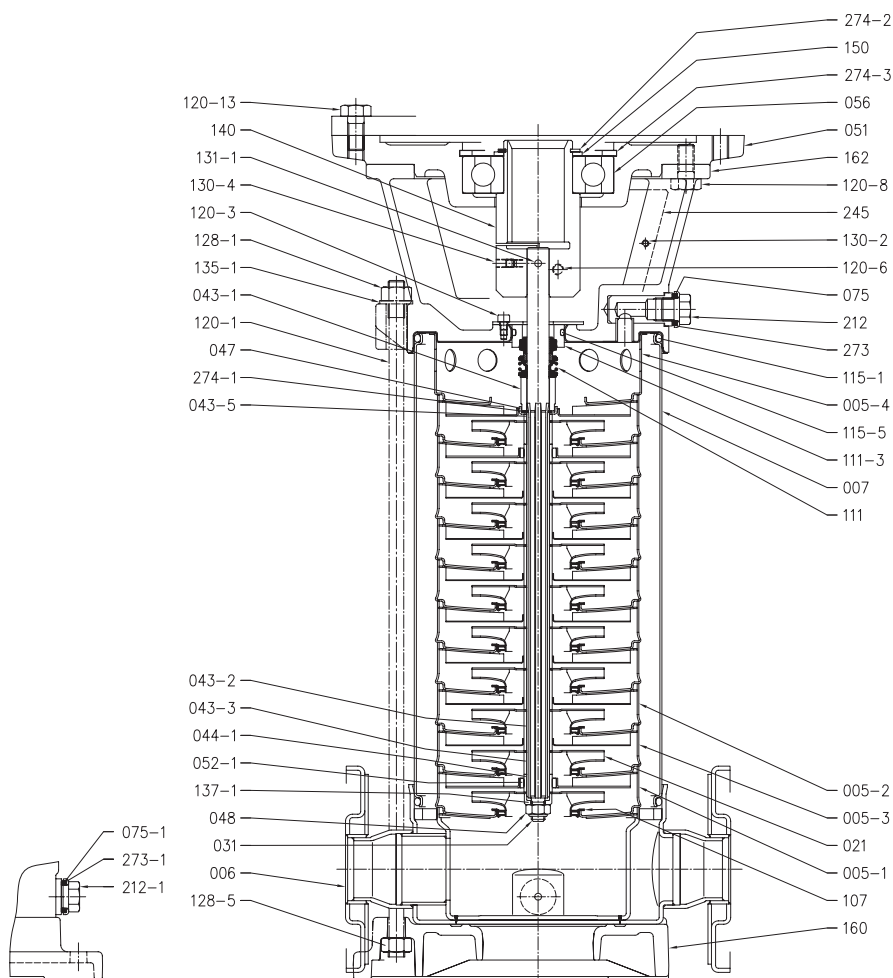
РАЗРЕЗ EVM(L) 3-18 Насос с одинарным шариковым подшипником
