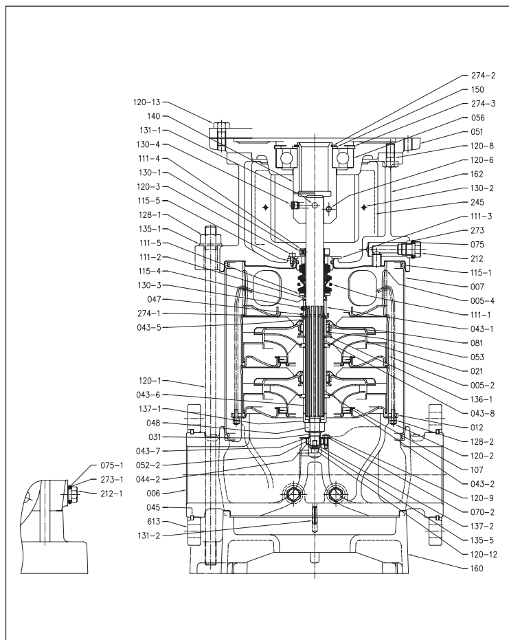
РАЗРЕЗ EVM(L) 45-64 Насос с одинарным шариковым подшипником
