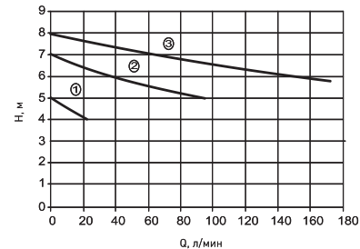
Рабочее поле для насоса С-32/8
