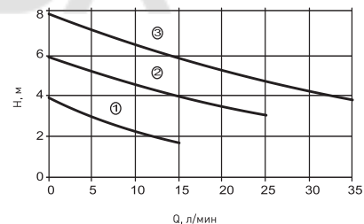
Рабочее поле для насоса С-25/8
