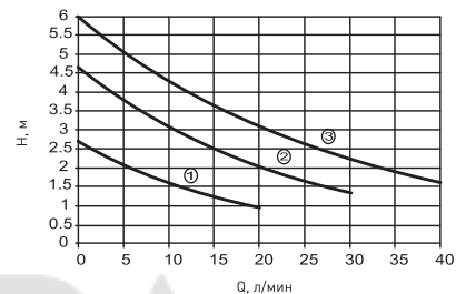
Рабочее поле для насосов С-25/6, С-32/6 и С-25/6-130
