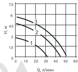
Напорно-расходные характеристики C-25/8
