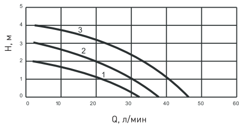
Напорно-расходные характеристики C-25/4, C-25/4-130 и C-32/4
