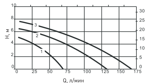
Напорно-расходные характеристики C-25/8N и C-32/8
