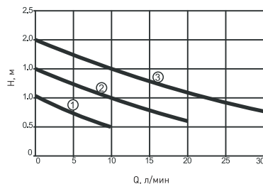
Напорно-расходные характеристики C-25/4, C-25/4-130 и C-32/4
