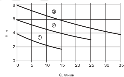
Напорно-расходные характеристики C-25/8N и C-32/8
