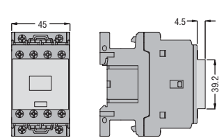
Крышка BFX80
