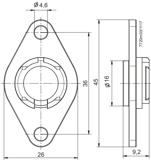
Фланец AGK42
