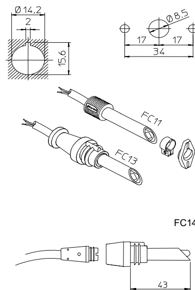
Рис. 5 – Установка датчиков FC1(1-3-4)
