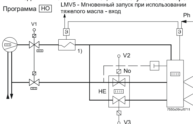
2-ступенчатая горелка
