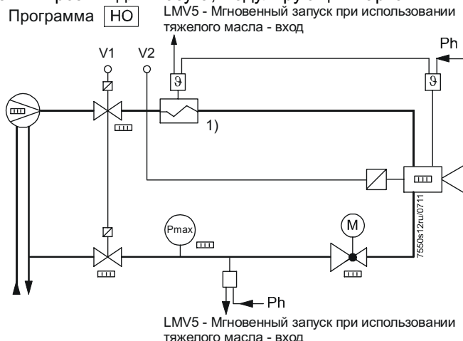
Модулированная горелка
