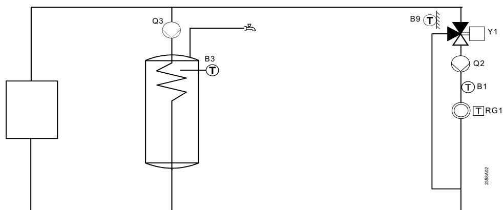
Стандартная схема
