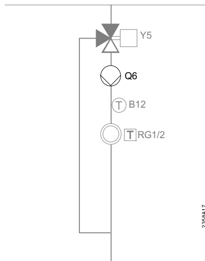
2-трубная система
