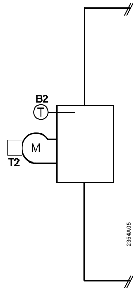
1-ступенчатая горелка
