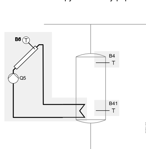
Аналогичная загрузка бака буфера
