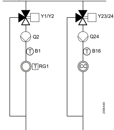
2-трубная система
