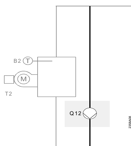
Насос на линии байпаса
