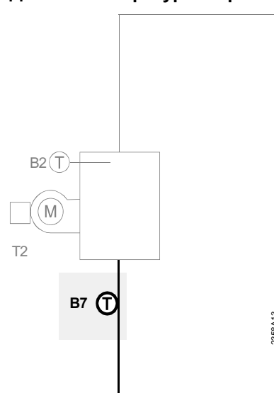
Датчик температуры обратной линии
