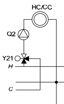
Пример: Подмес в 4-трубной системе
