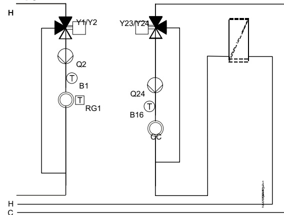
4-трубная система
