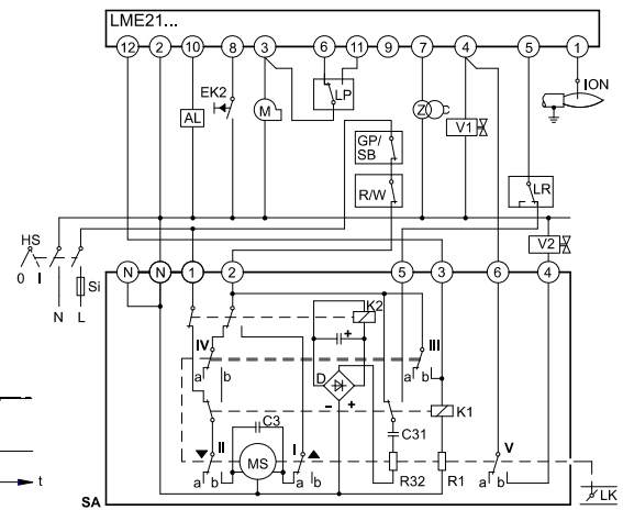
SQN91.140.../2-ступенчатое управление
