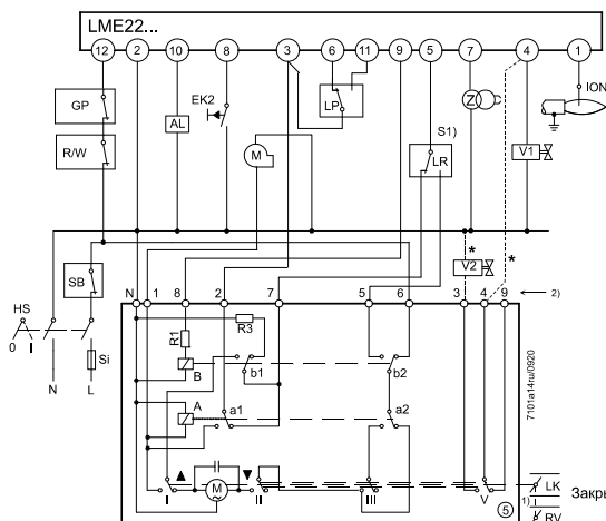
SQL3...151... или SQL3...251...
