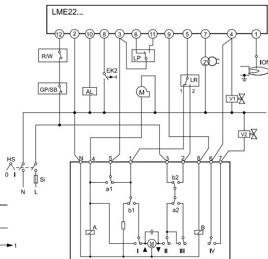
SQL7...424/2-ступенчатое управление 2-проводное управление
