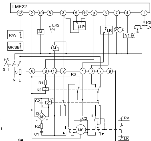
SQL90.220.../2-ступенчатое модулирующее управление
