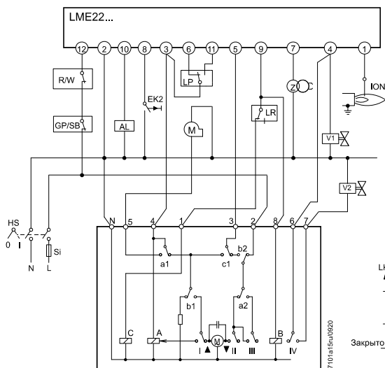
SQL7...454/2-ступенчатое управление 1-проводное управление
