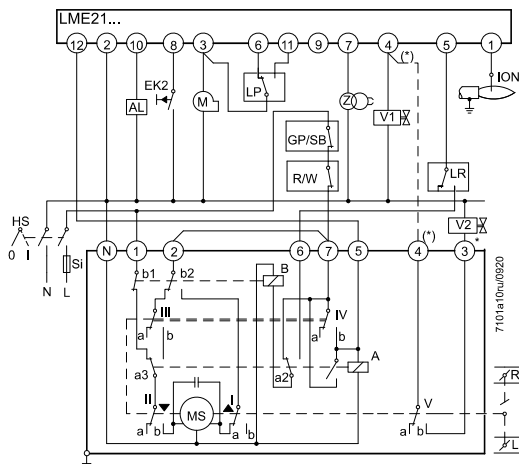
SQN3...121.../2-ступенчатое управление
