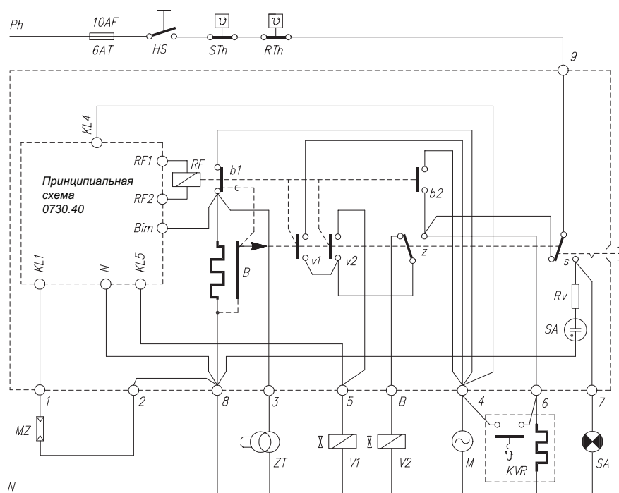
Электросхема TFI 836.3
