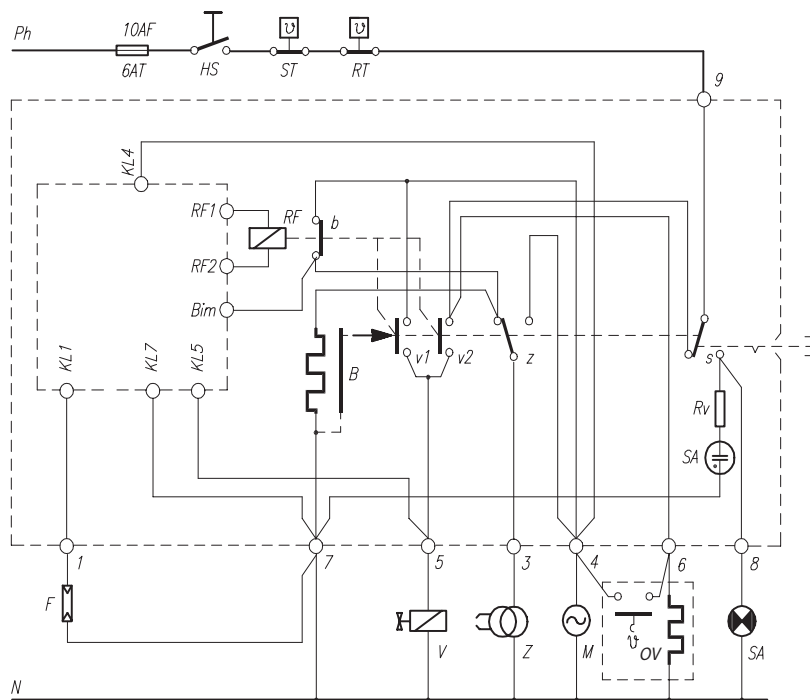
Электросхема TFI 974
