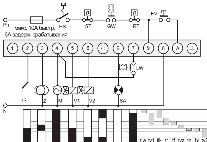
Без сервопривода воздушной заслонки для DMG 972 Mod.01
