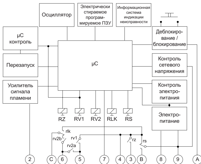
Блок-схема DMG 972
