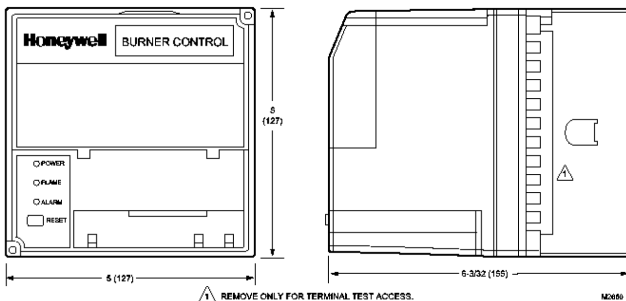
Рис. 1. Размеры EC7823 /RM7823 и суббазы Q7800A,B в дюймах (мм).
