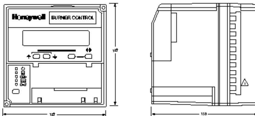
1 – СНИМАЕТСЯ ТОЛЬКО ДЛЯ ПРОВЕРКИ НАПЯЖЕНИЯ НА КЛЕММАХ
