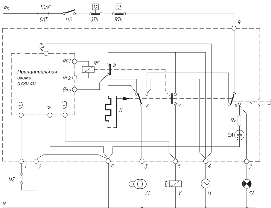
Электросхема TFI 830.3
