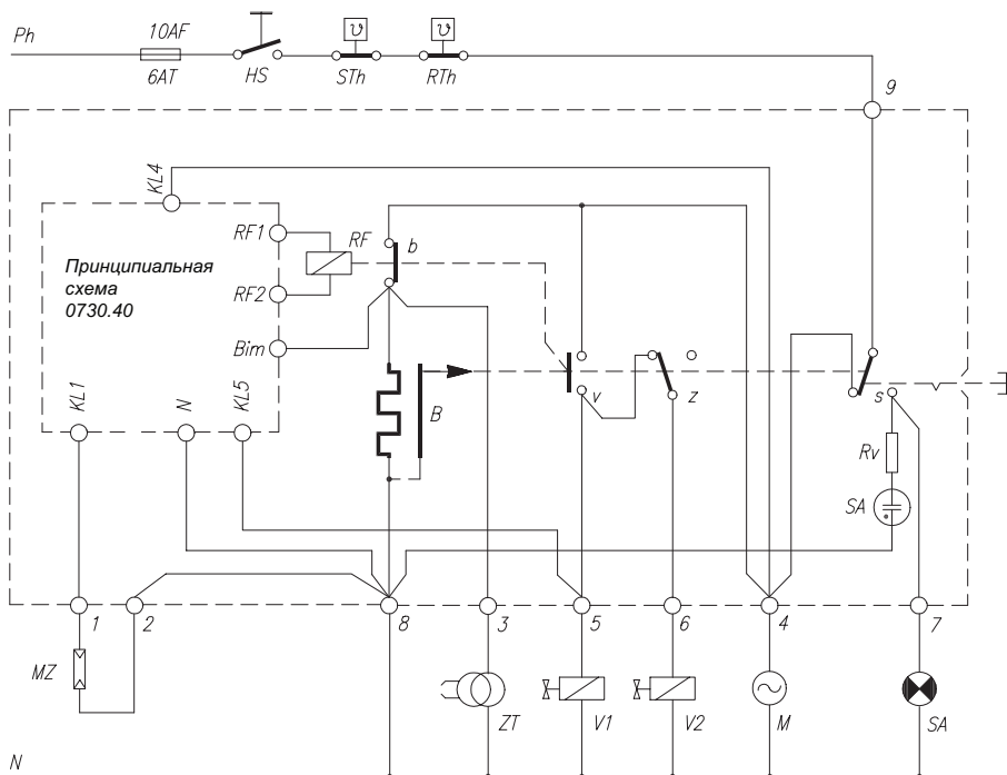
Электросхема TFI 832.3
