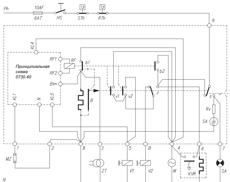
Электросхема TFI 836.3
