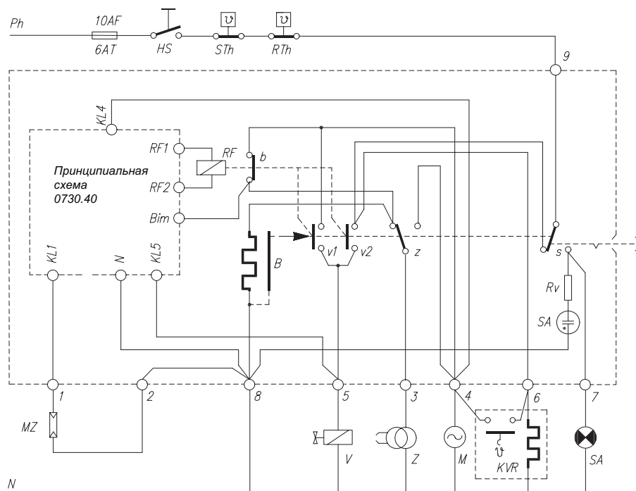
Электросхема TFI 834.3
