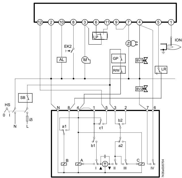
SQL7...244 / 2-х контурное регулирование
