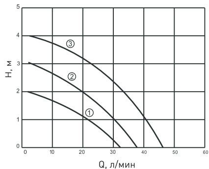
Рабочее поле для насосов C-25/4 и C-32/4
