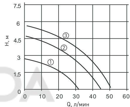
Рабочее поле для насосов C-25/6
