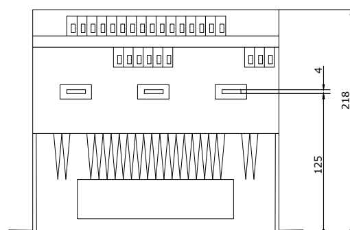
Вид снизу
