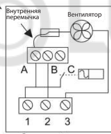
Питание платы управления
