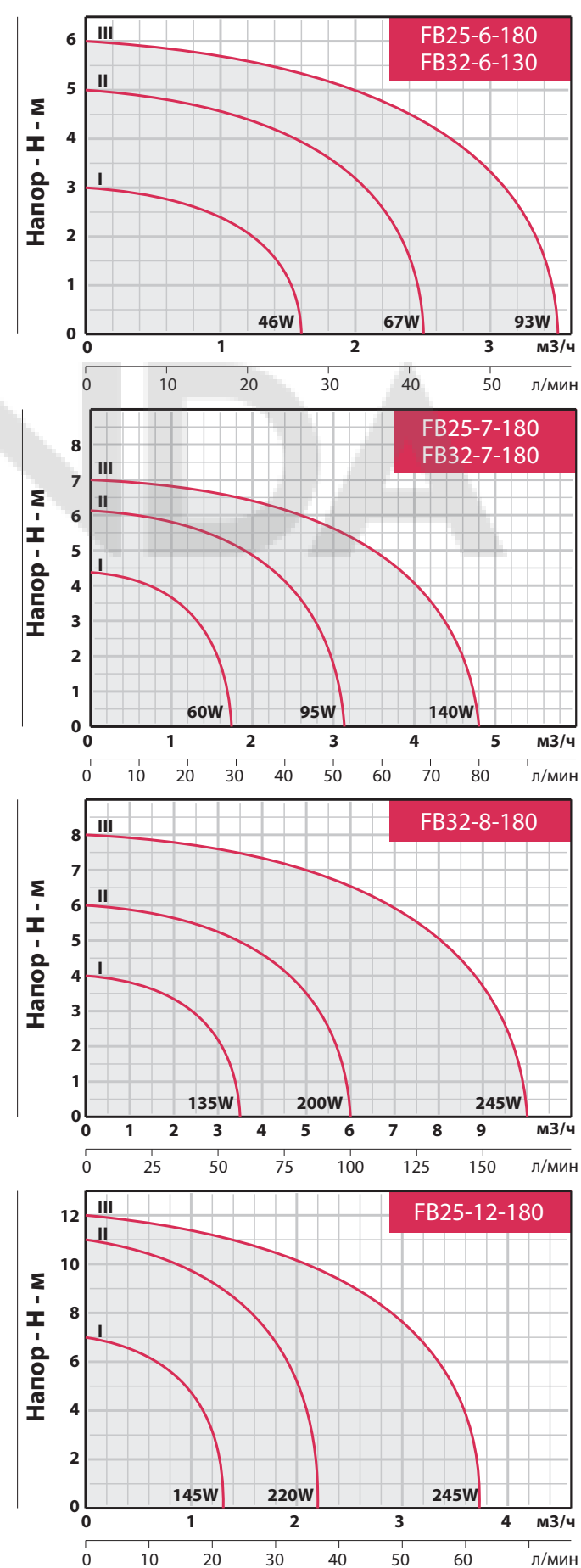
Кривая производительности
