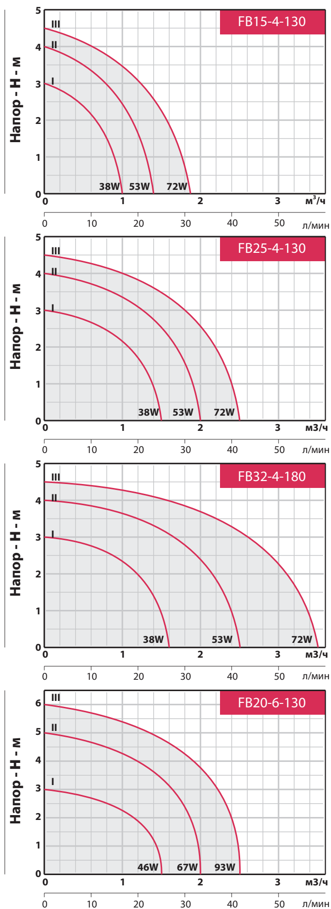
Кривая производительности
