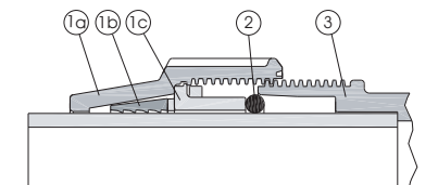
Water tightness of the fitting type DELT-ONE Ø 63, 75, 90, 110 mm Hydraulische Dichtigkeit des Fittings DELT-ONE Ø 63, 75, 90, 110 mm Гидравлическая непроницаемость переходника типа DELT-ONE Ø 63, 75, 90, 110 mm
