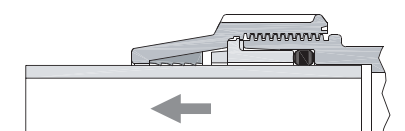
Water tightness of the fitting type DELT-ONE Ø 63, 75, 90, 110 mm Hydraulische Dichtigkeit des Fittings DELT-ONE Ø 63, 75, 90, 110 mm Гидравлическая непроницаемость переходника типа DELT-ONE Ø 63, 75, 90, 110 mm
