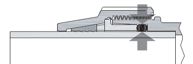
Water tightness of the fitting type DELT-ONE Ø 63, 75, 90, 110 mm Hydraulische Dichtigkeit des Fittings DELT-ONE Ø 63, 75, 90, 110 mm Гидравлическая непроницаемость переходника типа DELT-ONE Ø 63, 75, 90, 110 mm
