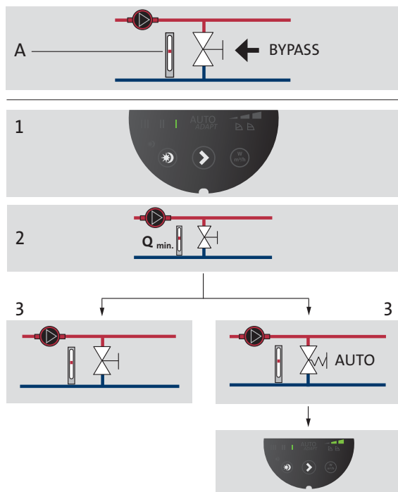
Рис. 23 Системы с перепускным клапаном
