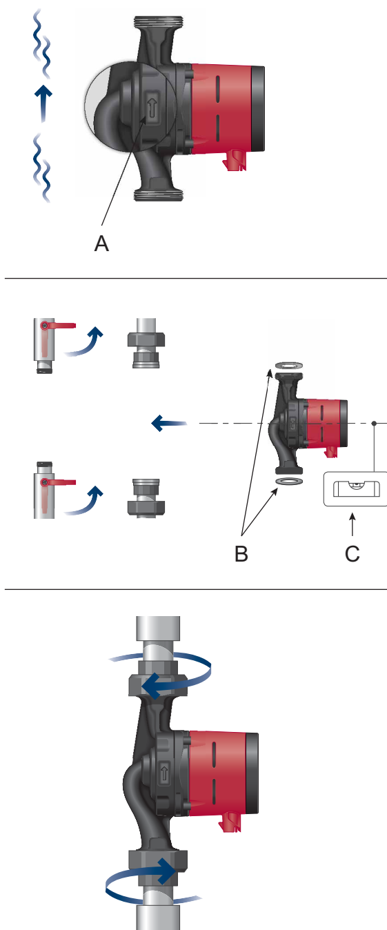
Рис. 3 Монтаж насоса GRUNDFOS ALPHA2
