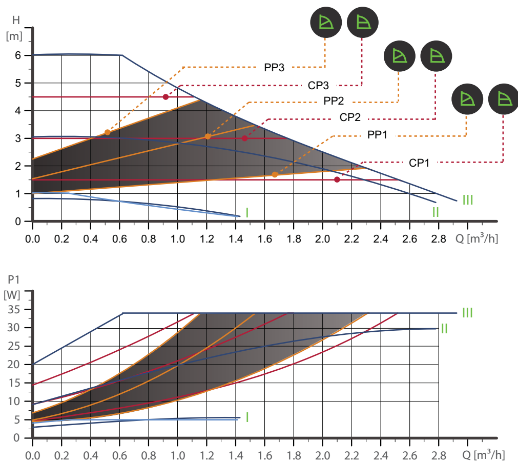
Рис. 34 ALPHA2 25-60 A
