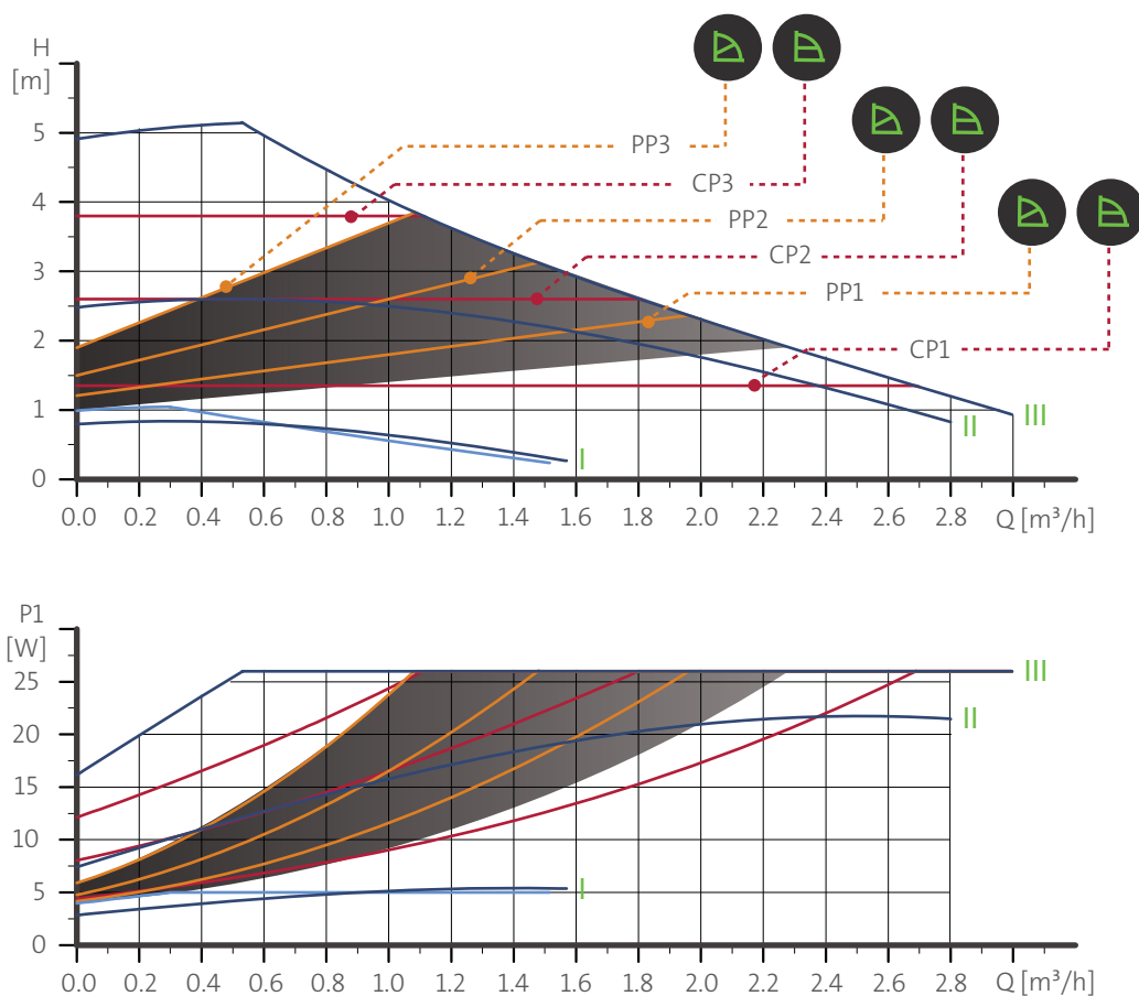
Рис. 31 ALPHA2 XX-50
