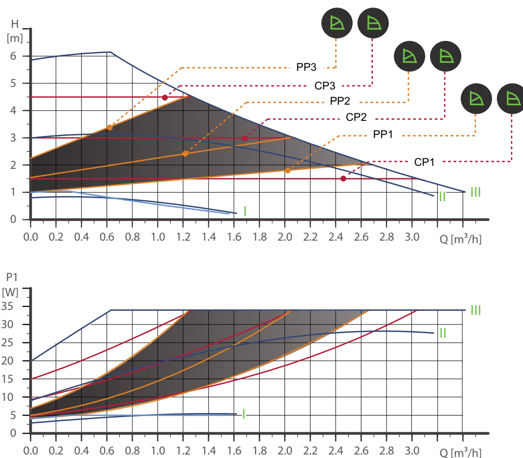
Рис. 32 ALPHA2 XX-60
