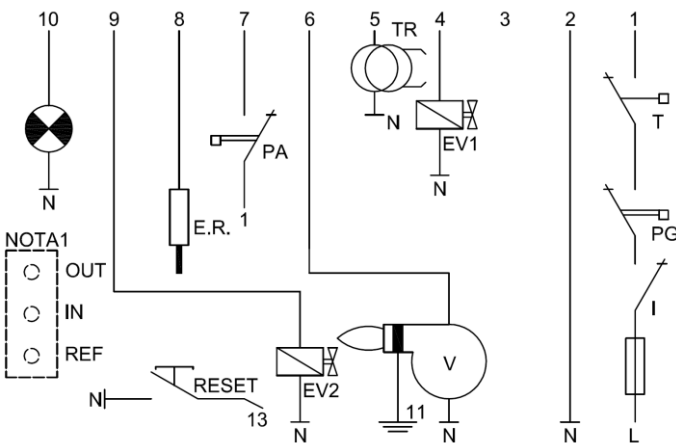
VM44G SENZA SERRANDA (opzione S)
