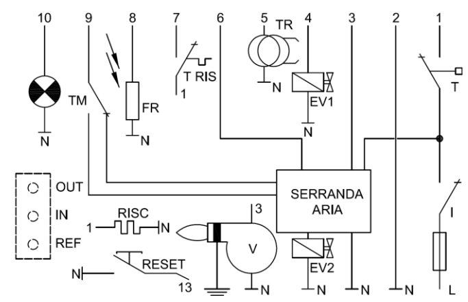
VM44O CON SERRANDA E TERMOSTATO DI MODULAZIONE A 2 FILI
